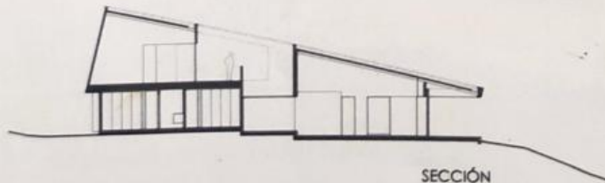
El esquema binuclear permitió el desarrollo de dos tipos de casas similares –una más compacta, otra más alargada– que se adaptan a la cambiante topografía del terreno.
